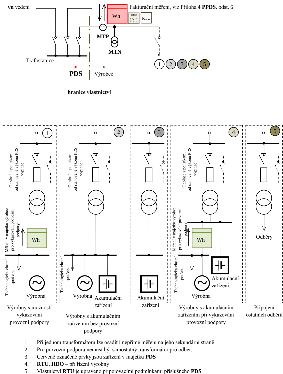
Obr. 19 Připojení výrobní a akumulačního zařízení zasmyčkováním do vn vedení DS
